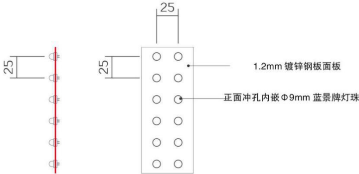
冲孔示意图 PUNCHING DIAGRAM
